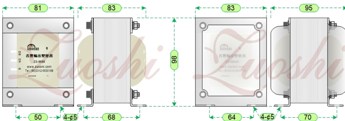
1: 立式安裝示意圖
