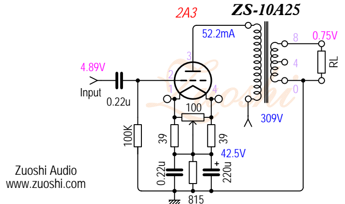
图1 ZS-10A25自给偏压测试电路
