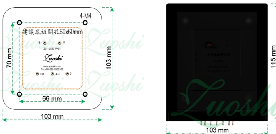
1: 全罩/密封安裝示意圖
